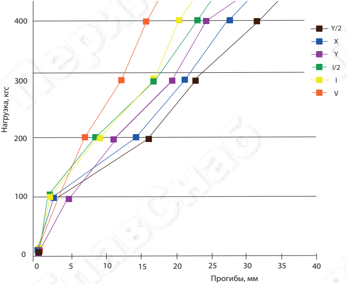
Зависимость прогибов концов консолей спайдеров от осевой силы:
