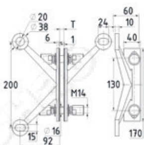
k290-Y R PSS AISI 304 k291-Y R PSS AISI 316 Y R -спайдер для установки на стеклянное ребро Предельные эксплуатационные нагрузки Fx -2500 Н (250кг), Fy -1500 Н (150кг)
