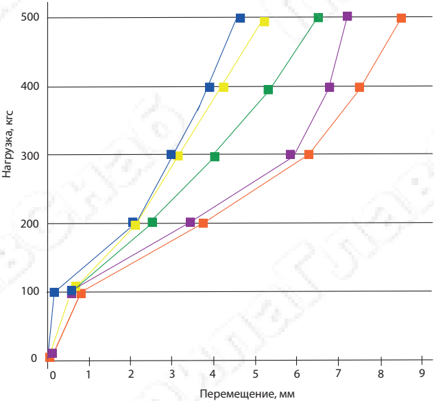
Графически зависимости перемещений концов консолей от величины растягивающей нагрузки:
