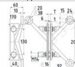
k290-Y/2 PSS AISI 304 k291-Y/2 PSS AISI 316 Y/2-спайдер для установки на стеклянное ребро Предельные эксплуатационные нагрузки Fx -2500 Н (250кг), Fy -1500 Н (150кг)
