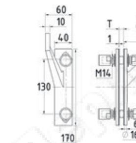
k290-I PSS AISI 304 k291-I PSS AISI 316 I-спайдер для установки на стеклянное ребро Предельные эксплуатационные нагрузки Fx -2500 Н (250кг), Fy -1500 Н (150кг)
