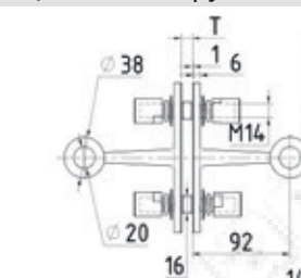
k290-I/2 PSS AISI 304 k291-I/2 PSS AISI 316 I/2-спайдер для установки на стеклянное ребро Предельные эксплуатационные нагрузки Fx -2500 Н (250кг), Fy -1500 Н (150кг)
