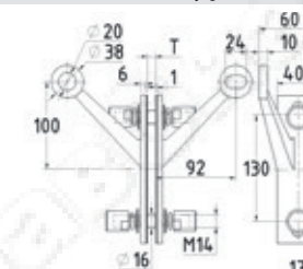
k290-V/2L PSS AISI 304 k291-V/2L PSS AISI 316 V/2L-спайдер для установки на стеклянное ребро Предельные эксплуатационные нагрузки Fx -2500 Н (250кг), Fy -1500 Н (150кг)
