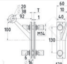
k290-V/2R PSS AISI 304 k291-V/2R PSS AISI 316 V/2R-спайдер для установки на стеклянное ребро Предельные эксплуатационные нагрузки Fx -2500 Н (250кг), Fy -1500 Н (150кг)
