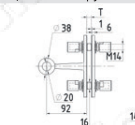
k290-I/2 PSS AISI 304 k291-I/2 PSS AISI 316 I/2-спайдер для установки на стеклянное ребро Предельные эксплуатационные нагрузки Fx -2500 Н (250кг), Fy -1500 Н (150кг)
